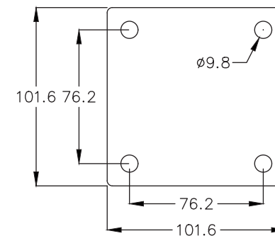
30系列 9# 平板 30 Series 9# Top Plate
