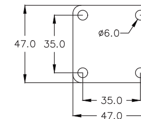
15系列珠皿平板尺寸 15 Series Top Plate
