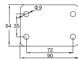
30系列 7# 平板 30 Series 7# Top Plate
