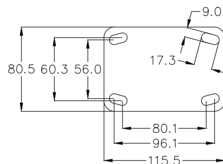
32系列1#平板尺寸 32Series 1#Top Plate
