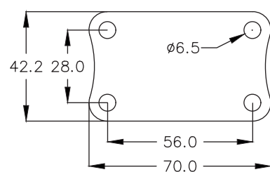
107系列平板尺寸 107 Series Top Plate
