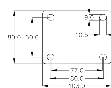
37系列平板尺寸 37 Series Top Plate
