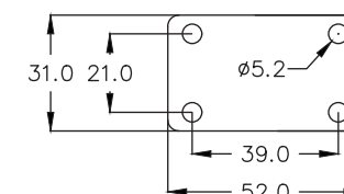
15系列平板尺寸 15 Series Top Plate
