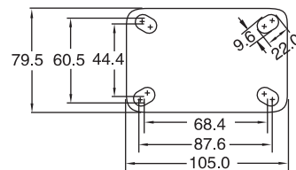
30系列4#平板 30 Series 4# Top Plate
