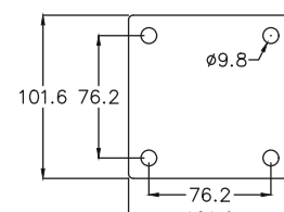
30系列 9# 平板 30 Series 9# Top Plate
