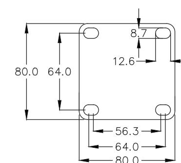
30系列 6# 平板 30 Series 6# Top Plate
