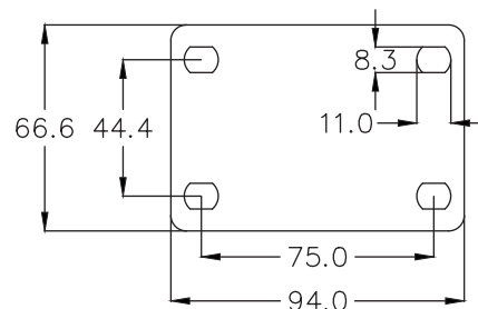
24系列平板尺寸 24 Series Top Plate
