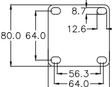
30系列 6# 平板 30 Series 6# Top Plate
