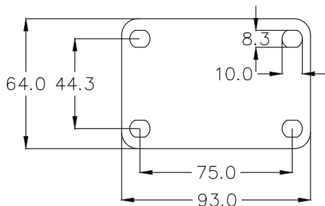
22系列平板尺寸 22 Series Top Plate
