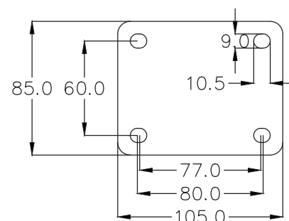
32系列2#平板尺寸 32Series 2#Top Plate
