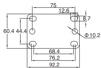
30系列 2# 平板 30 Series 2# Top Plate
