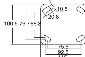
30系列 8# 平板 30 Series 8# Top Plate
