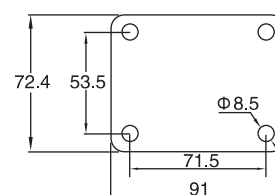
30系列 10# 平板 30 Series 10# Top Plate
