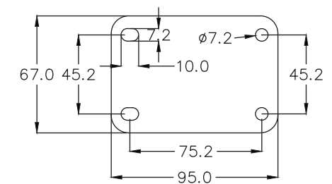
102系列平板尺寸 102 Series Top Plate
