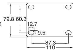
30系列3#平板 30 Series 3# Top Plate
